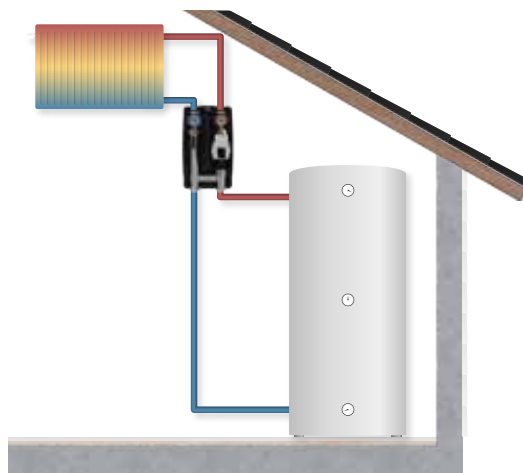
LK 861 H 125 - Gruppo pompa ideale per gli impianti di riscaldamento ad alimentazione diretta.
