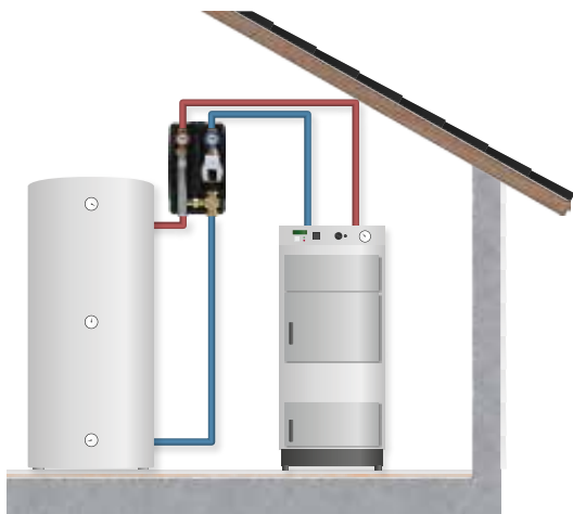
LK 864 H 125 - Gruppo pompa con una valvola anticondensa LK 823 ThermoVar®. Il gruppo pompa è progettato per garantire un'ottimale stratificazione della temperatura nel sistema di accumulo e, contemporaneamente, garantire una elevata temperatura di ritorno verso la caldaia. Questo aumenta l'efficienza del sistema.
