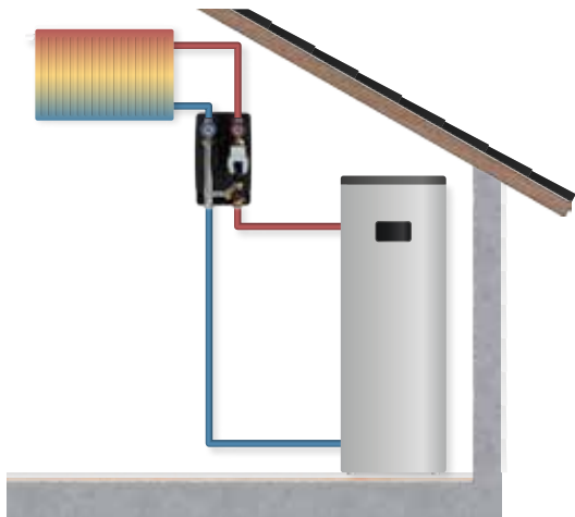
LK 862 H 125 - Gruppo pompa ideale per gli impianti di riscaldamento ad alimentazione con valvola miscelatrice. È inclusa una valvola miscelatrice a tre vie.
