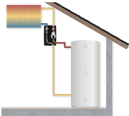
LK 866 H 125 - Gruppo pompa con una valvola miscelatrice a quattro vie, LK 841 ThermoMix®. Il gruppo pompa è destinato per impianti di riscaldamento dove si desidera una elevata temperatura dell'acqua di ritorno verso la caldaia.
