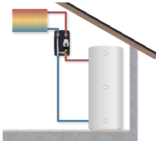
LK 863 H 125 - Gruppo pompa ideale per gli impianti di riscaldamento ad alimentazione con valvola miscelatrice. È inclusa una valvola miscelatrice termica. LK 551 HydroMix ha un elemento termostatico che regola l'alimentazione e il ritorno per raggiungere la temperatura di mandata desiderata.
