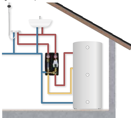
LK 865 H 125 - Gruppo completo per la circolazione dell'acqua calda sanitaria. Comprende una valvola miscelatrice, croce, pompa di ricircolo, isolamento, kit di connessione e tre valvole di ritegno. LK 551 HydroMix valvola miscelatrice ha un elemento termostatico per regolare la temperatura dell'acqua al valore desiderato.
