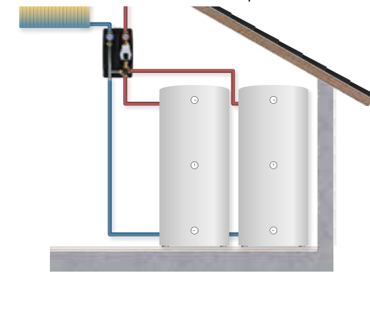
LK 867 H 125 - Gruppo pompa con una valvola miscelatrice a quattro vie, LK 830 ThermoMix® B. Il gruppo pompa è dotato di una valvola miscelatrice bivalente a quattro vie progettata per impianti di riscaldamento, dove l'energia viene prelevata da due unità di riscaldamento collegate in serie o in parallelo, oppure per sistemi di accumulo dove l'energia viene prelevata da due livelli. Il gruppo pompa deve essere equipaggiato con un'unità di controllo automatico per garantire che venga sempre data priorità alla fonte di calore più favorevole.
