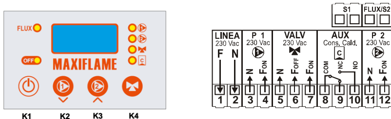
Fig. 1 Aspetto esterno e Schema dei collegamenti elettrici
